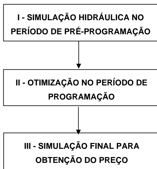
Figura I.2 - Módulos em que se subdivide o Modelo DESSEM
