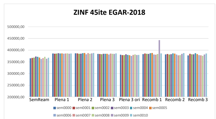
Figura 2.4 – Comportamento do ZINF, médio e por semente inicial.
