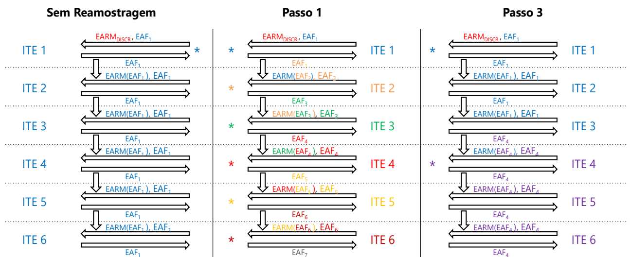
Figura 2.3 – Utilização das amostras de afluições na recursão backward e na simulação forward Momento de reamostragem forward .
