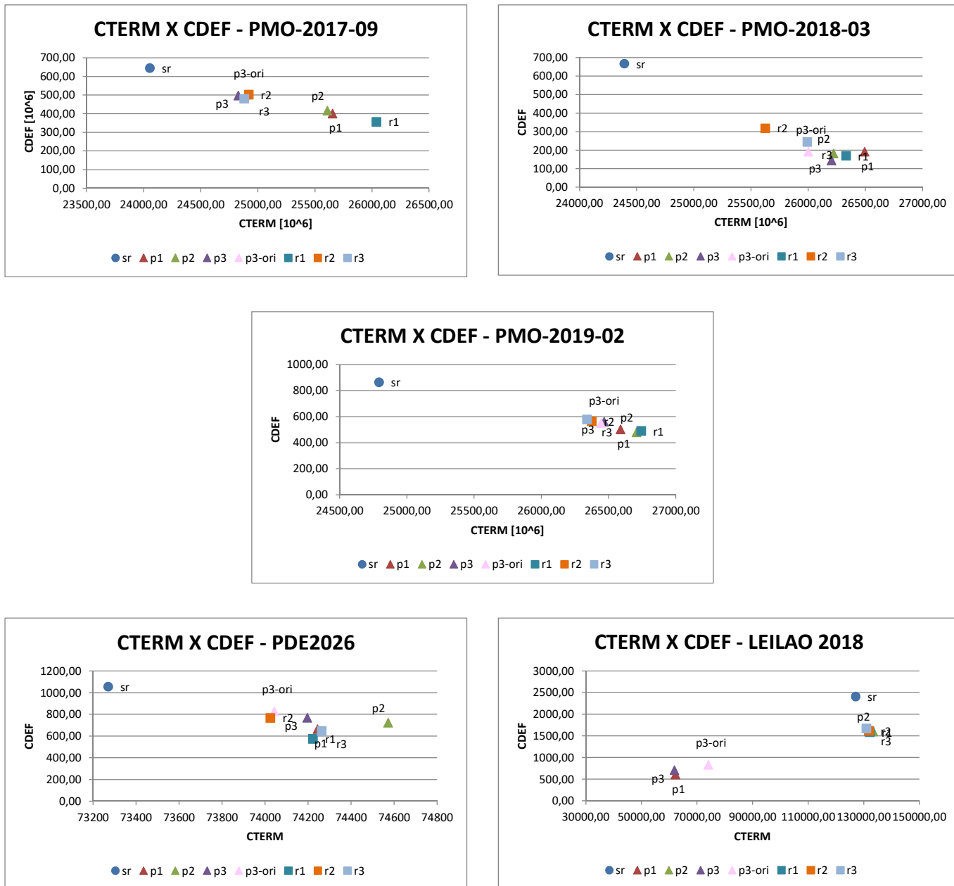
Figura 2.5 – Análise de trade-off entre o custo esperado de geração térmica e o custo esperado de déficit.
