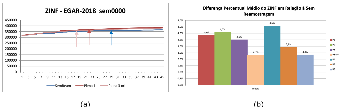
Figura 3.1 – Evolução do ZINF ao longo das iterações (a) e \Delta ZINF (%) em relação ao caso sem reamostragem (b).
