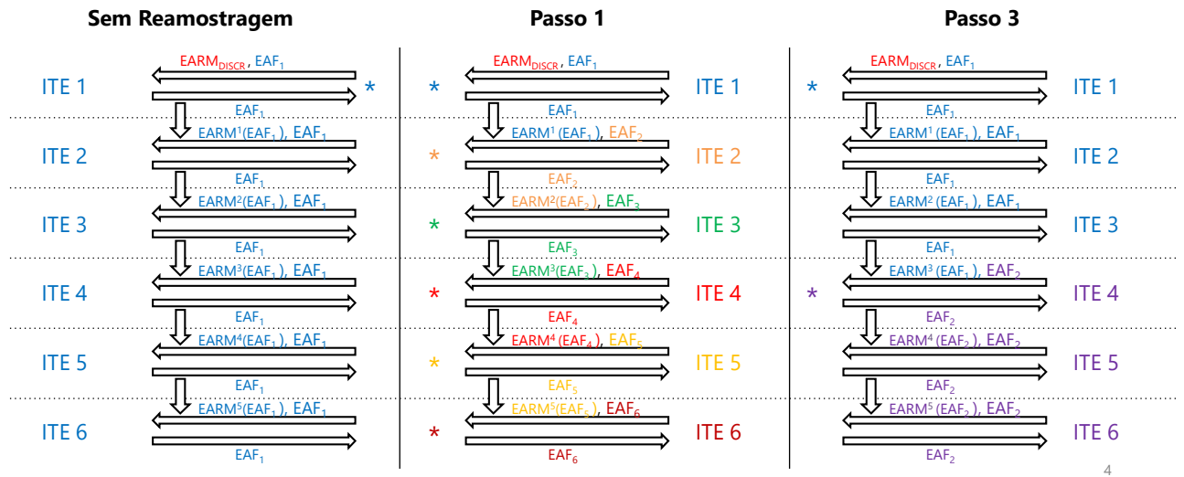
Figura 2.2 – Utilização das amostras de aflúências na recursão backward e na simulação forward Momento de reamostragem backward .
