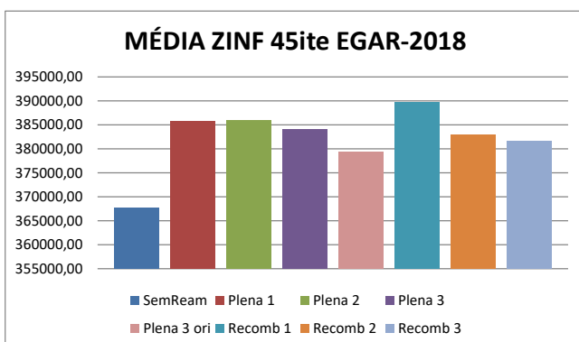
Figura 2.4 – Comportamento do ZINF, médio e por semente inicial.
