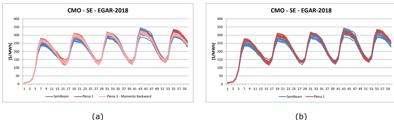
Figura 2.6 – Comportamento do valor esperado do CMO ao longo do horizonte de planejamento.
