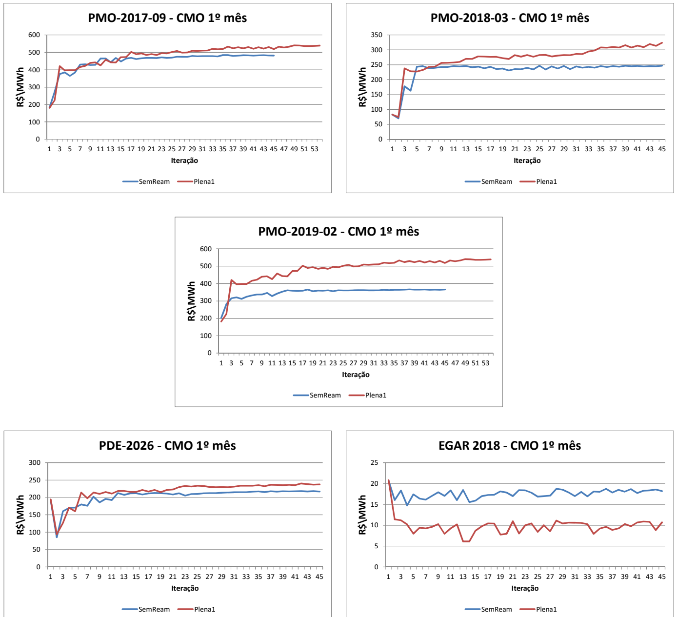
Figura 3.3 – Valor esperado do CMO em cada iteração do algoritmo de PDDE.
