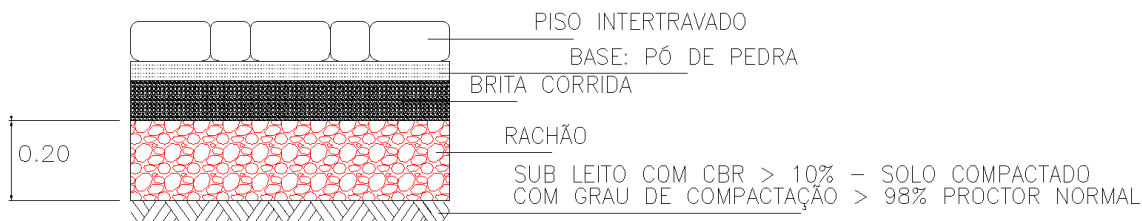
Figura 3: Perfil transversal das camadas estruturais da pavimentação.
