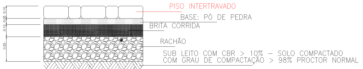
Figura 3: Perfil transversal das camadas estruturais da pavimentação.
