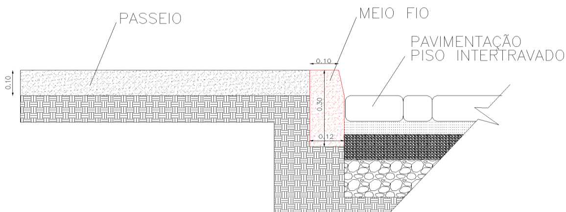
Figura 3: Desenho esquemático do perfil do meio-fio com as camadas de pista e passeio.
