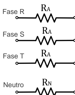
Figura 2 – Diagrama esquemático das Resistências de Cintilação
