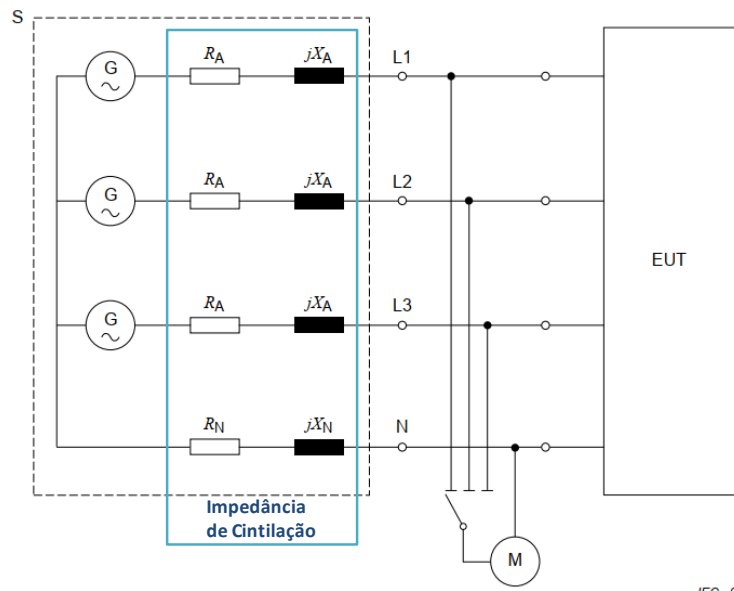
Figura 1 – Configuração do ensaio de avaliação de cintilação, adaptado de IEC 61000-3-3. Onde G= Fonte CA, M= medição, EUT= Equipment under Test .
