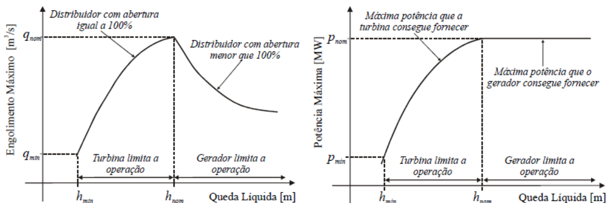
Figura 6-25 - Engolimento máximo e potência máxima de um conjunto turbina/gerador em função da altura de queda líquida.
