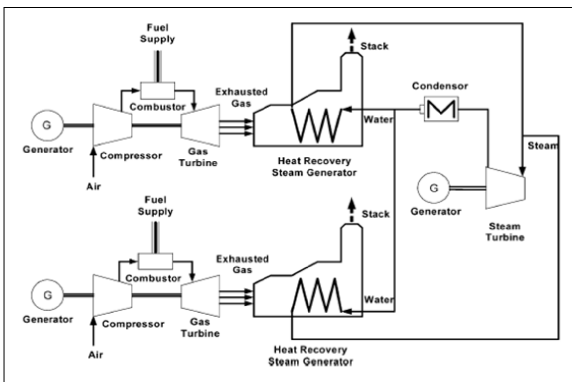
Figura 7-3 - Esquema de uma usina térmica a ciclo combinado com duas turbinas a gás e uma turbina a vapor.
