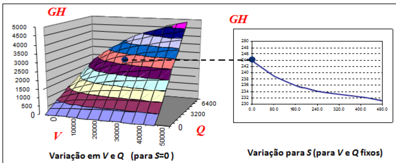
Figura 6-20 - Gráfico da função de produção exata (FPH) de uma usina hidrelétrica.
