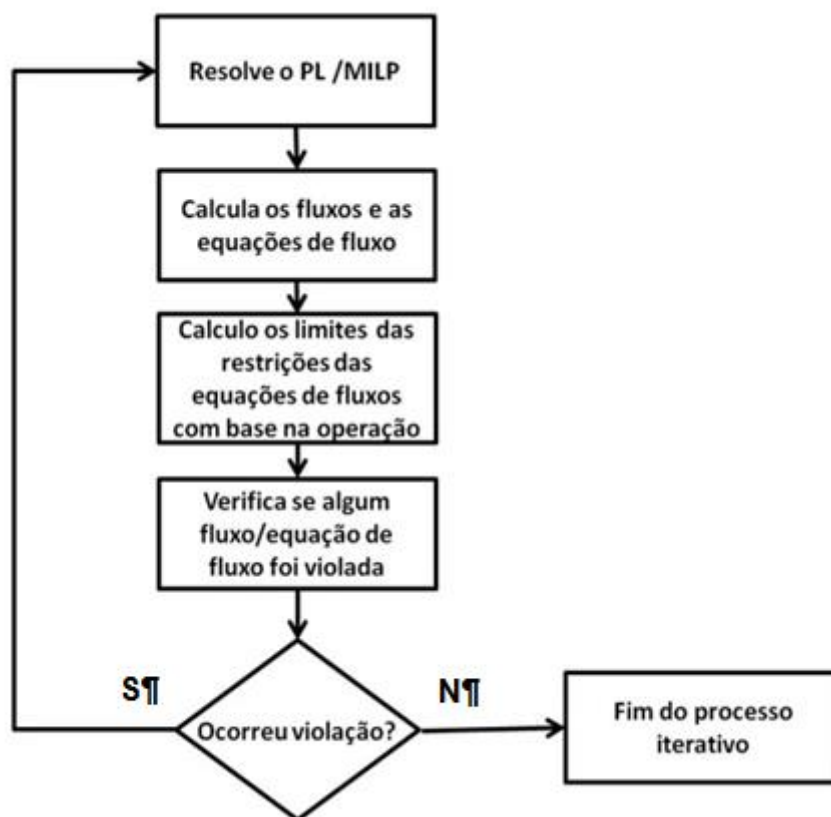
Figura 18-2 - Fluxograma para considerar limites das Restrições de Segurança Elétrica definidos por Tabelas.
