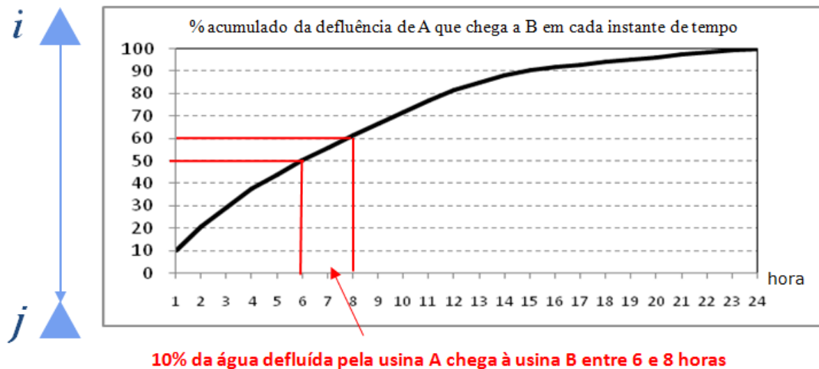
Figura 6-13 - Exemplo de uma curva de propagação de tempo de viagem da usina de montante i até a usina de jusante j
