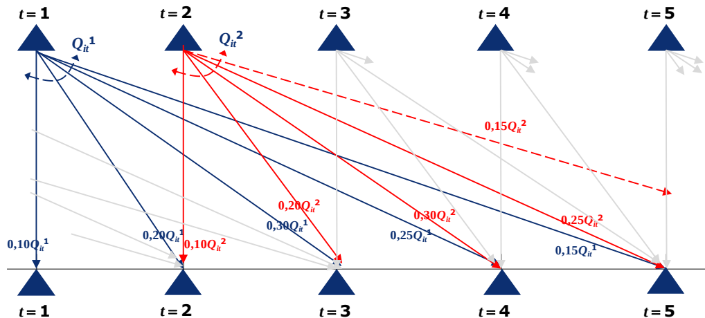
Figura 6-14 - Esquema de saída da usina de montante e chegada na usina de jusante para a modelagem de tempo de viagem por curva de propagação.
