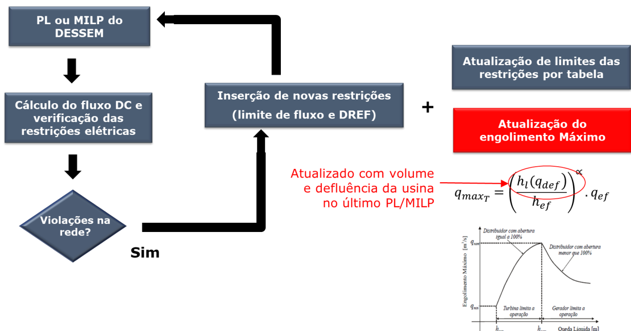
Figura 6.2 - Processo iterativo de cálculo do engolimento máximo, a cada recursão de resolução do PL ou MILP do modelo DESSEM
