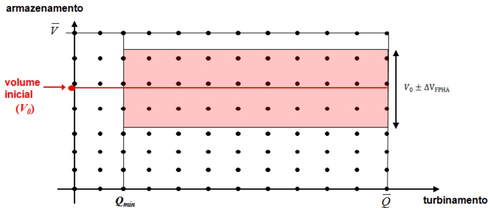
Figura 6-21 - Exemplo de janela de discretização para modelagem da FPHA.
