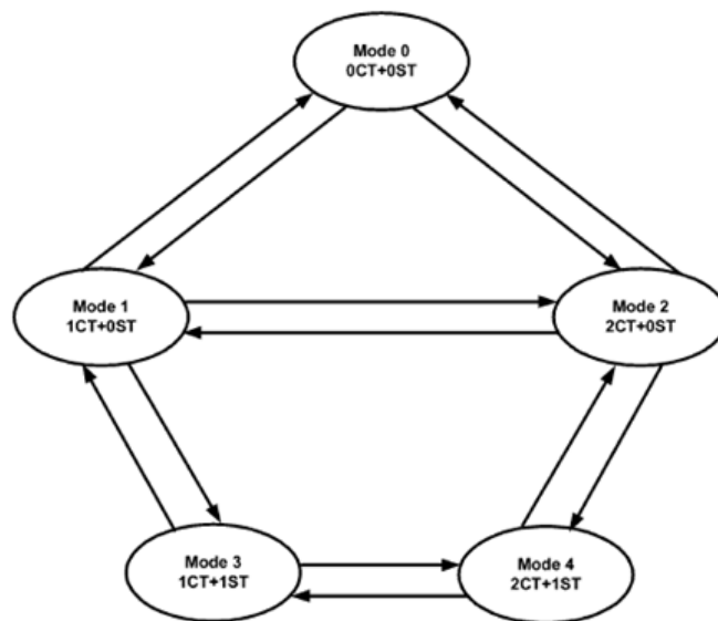
Figura 7-4 - Esquema ilustrativo das possíveis configurações operativas de uma usina térmica a ciclo combinado, e a transição entre elas (Fonte: Erro! Fonte de referência não encontrada.).
