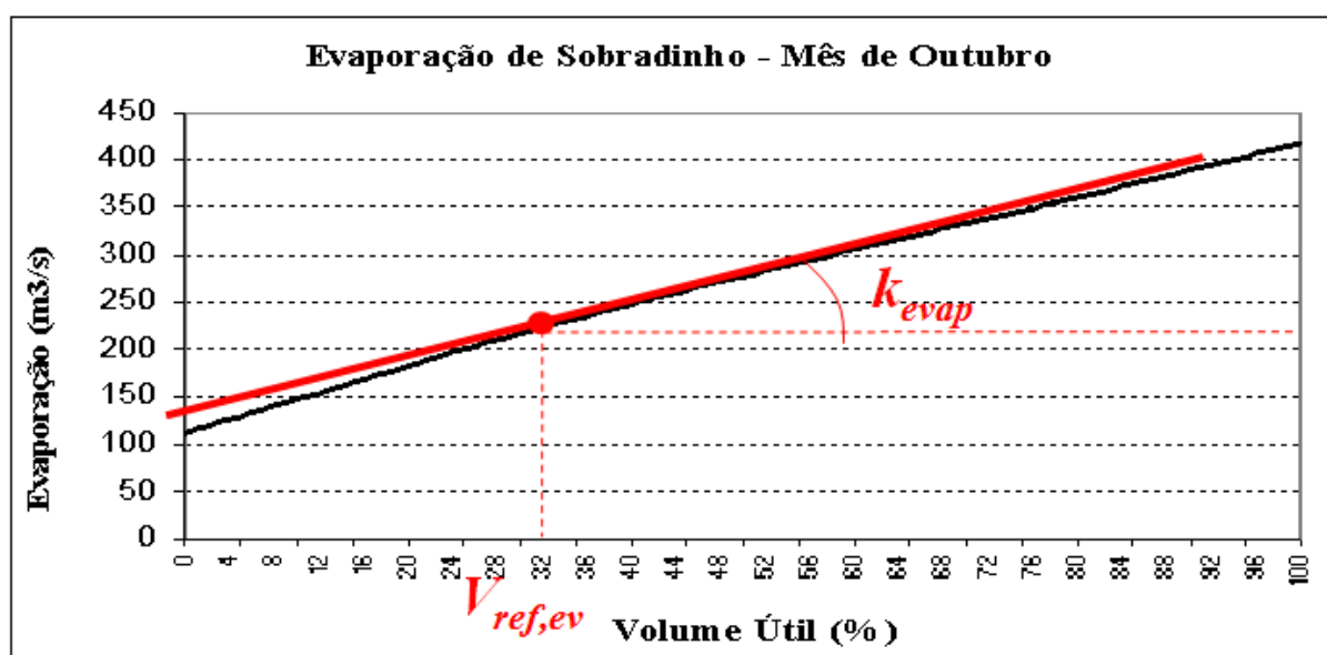
Figura 6-17 - Exemplo de modelo linear para a evaporação no reservatório de Sobradinho.
