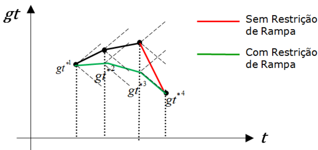
Figura 7-3 - Esquema ilustrativo do efeito das restrições de rampa de geração na operação de uma unidade térmica.
