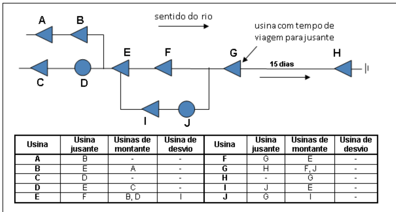
Figura 6-2 - Exemplo ilustrativo de uma cascata de usinas hidrelétricas contendo usinas de jusante, usinas de desvio e usina de jusante com tempo de viagem da água.
