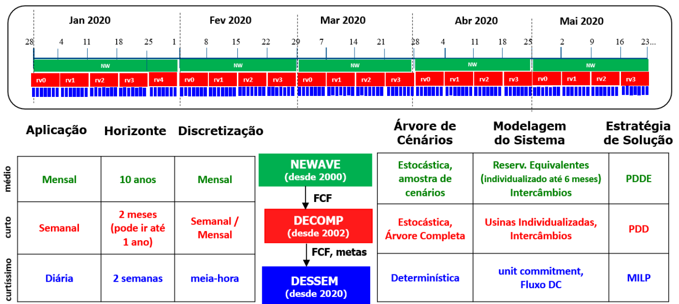
Figura 3-1 - Processo de planejamento da operação e estabelecimento do preço no mercado de curto prazo para o Sistema Interligado Nacional Brasileiro (SIN) utilizando os modelos desenvolvidos pelo CEPEL. O modelo DESSEM passou a ser utilizado a partir de janeiro de 2020 pelo ONS para despacho pelo ONS, e a partir de 2021 para formação de preço pela CCEE.
