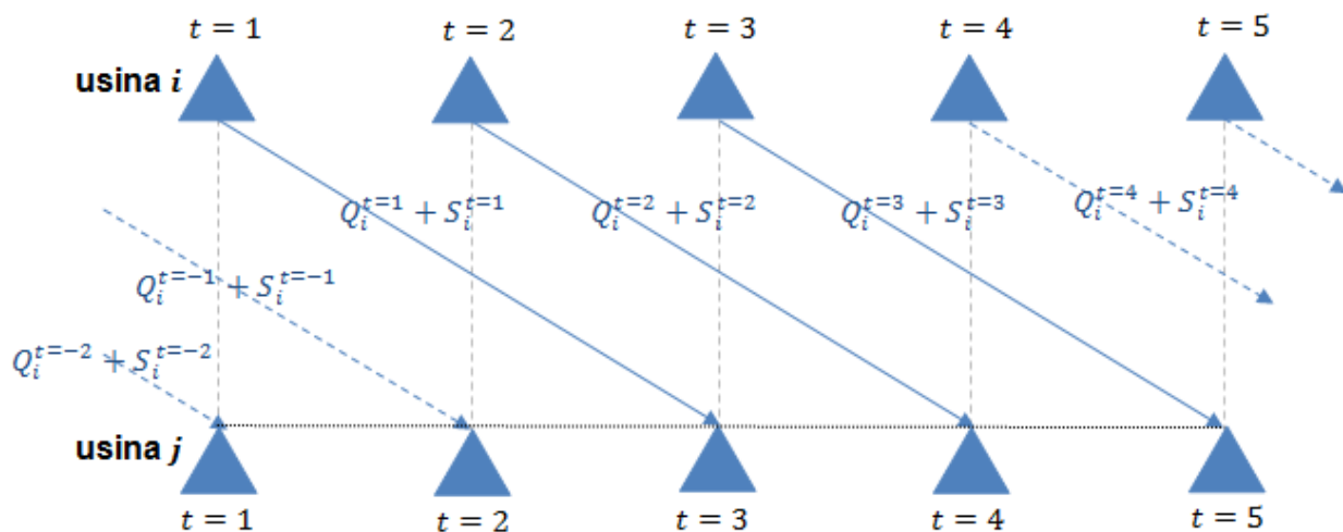
Figura 6-12 - Exemplo da modelagem por translação do tempo de viagem entre as usinas i e j , para um tempo de viagem de 2 horas.
