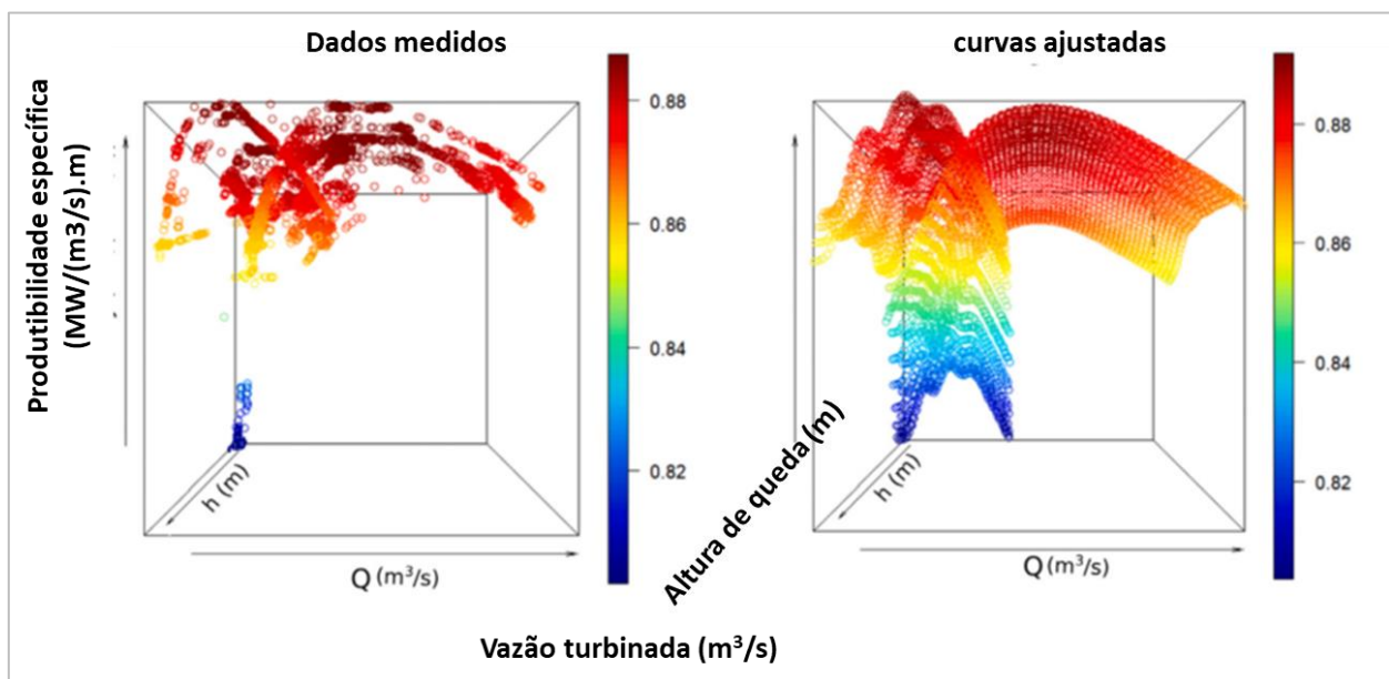
Figura 6-19 – Dados medidos e curva ajustada para a produtividade específica das usinas variável com a altura de queda e a vazão.
