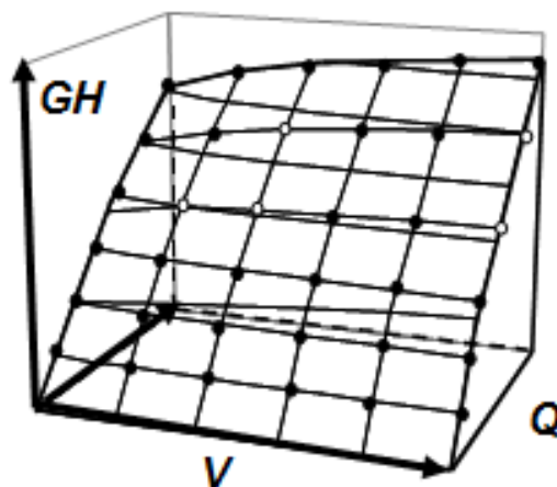
Figura 6-22 - Envoltória convexa da função FPH(V, Q) , para uma janela e grade de discretização definida para as variáveis V e Q .
