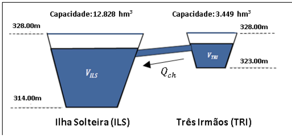
Figura 6-9 - Esquema ilustrativo de um Canal entre usinas hidrelétricas.
