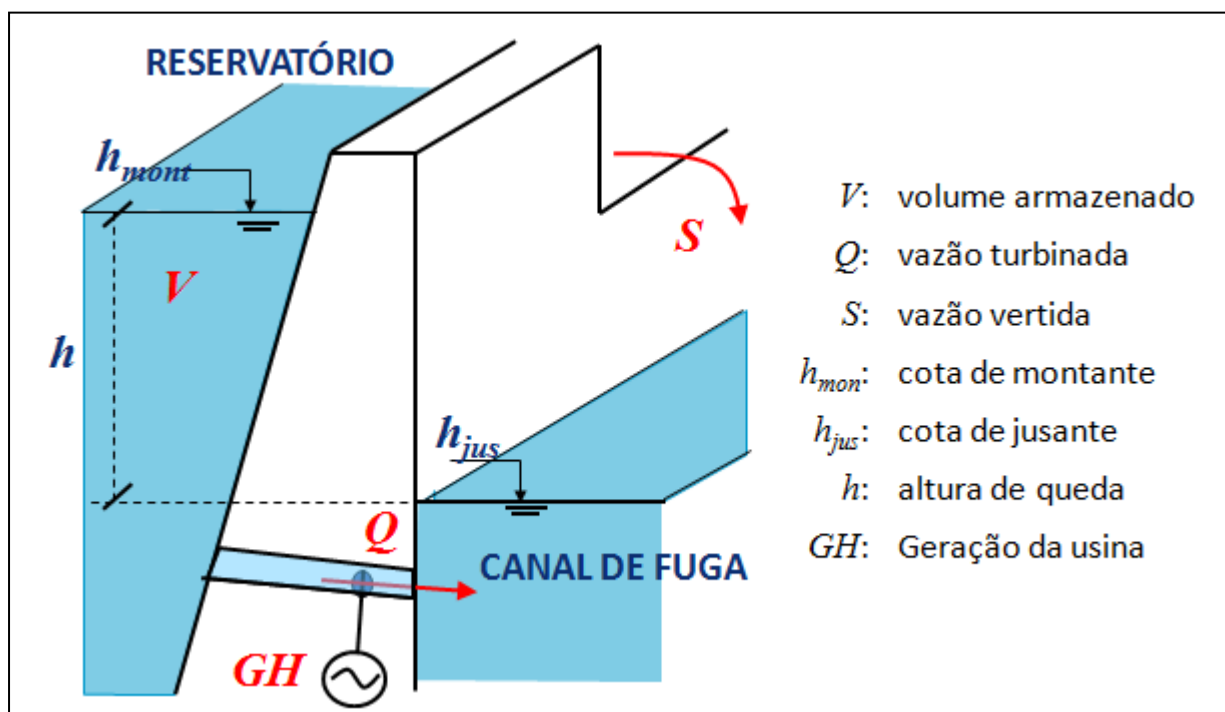
Figura 6-1--Representação esquemática de uma usina hidrelétrica e suas principais variáveis operativas.
