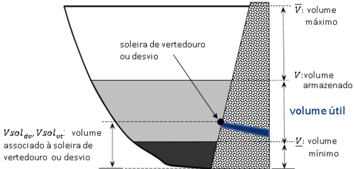
Figura 6-3 - Esquema ilustrativo de um reservatório.
