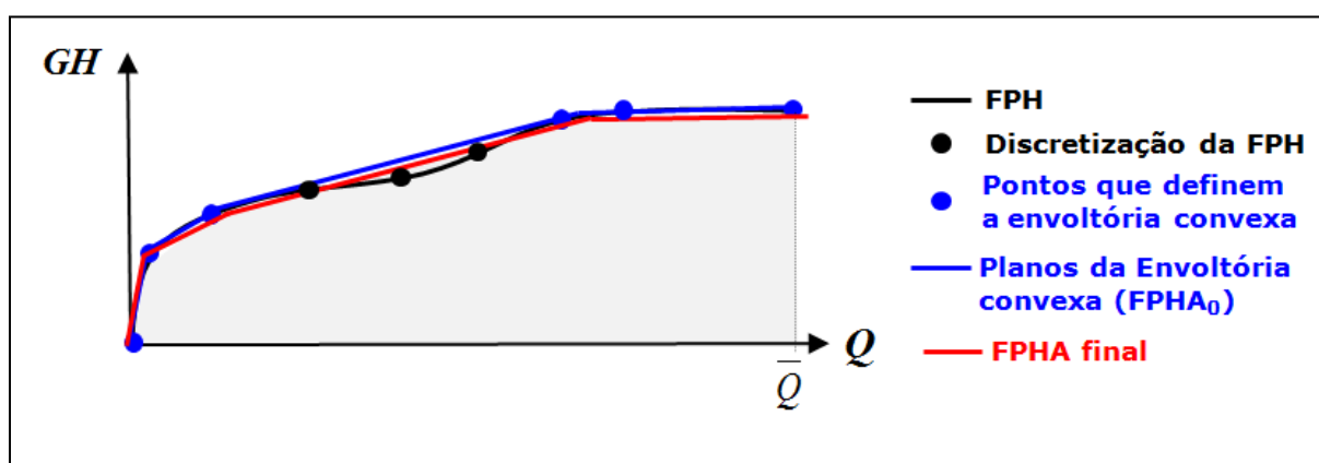
Figura 6-23 - Esquema ilustrativo da regressão feita para minimizar os desvios entre a FPH e a FPHA, após construção da envoltória convexa no plano (V, Q) .
