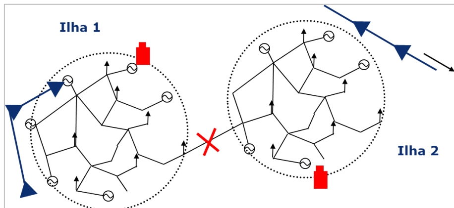
Figura 11.1 - Exemplo da formação de ilhas elétricas na rede elétrica, após desligamento de um circuito.
