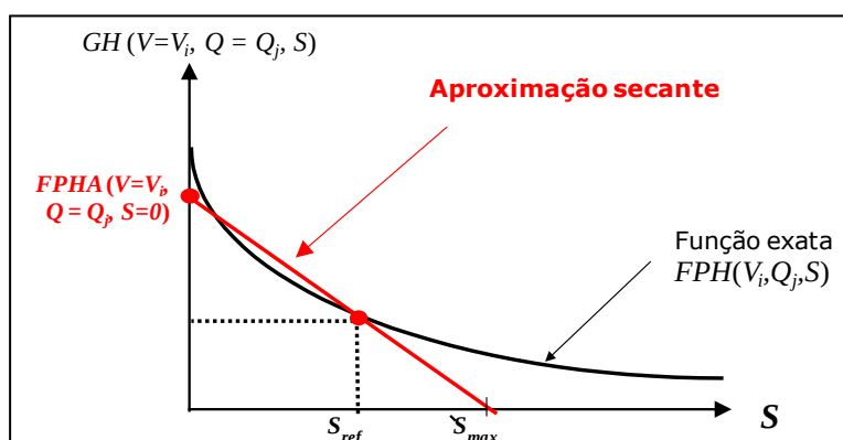
Figura 6-24 - Esquema ilustrativo da regressão feita para minimizar os desvios entre a FPH e a FPFA, após construção da envoltória convexa no plano (V,Q) .
