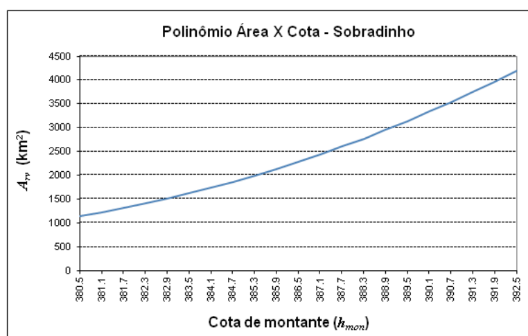
Figura 6-5 - Exemplo do polinômio cota-área da usina de Sobradinho
