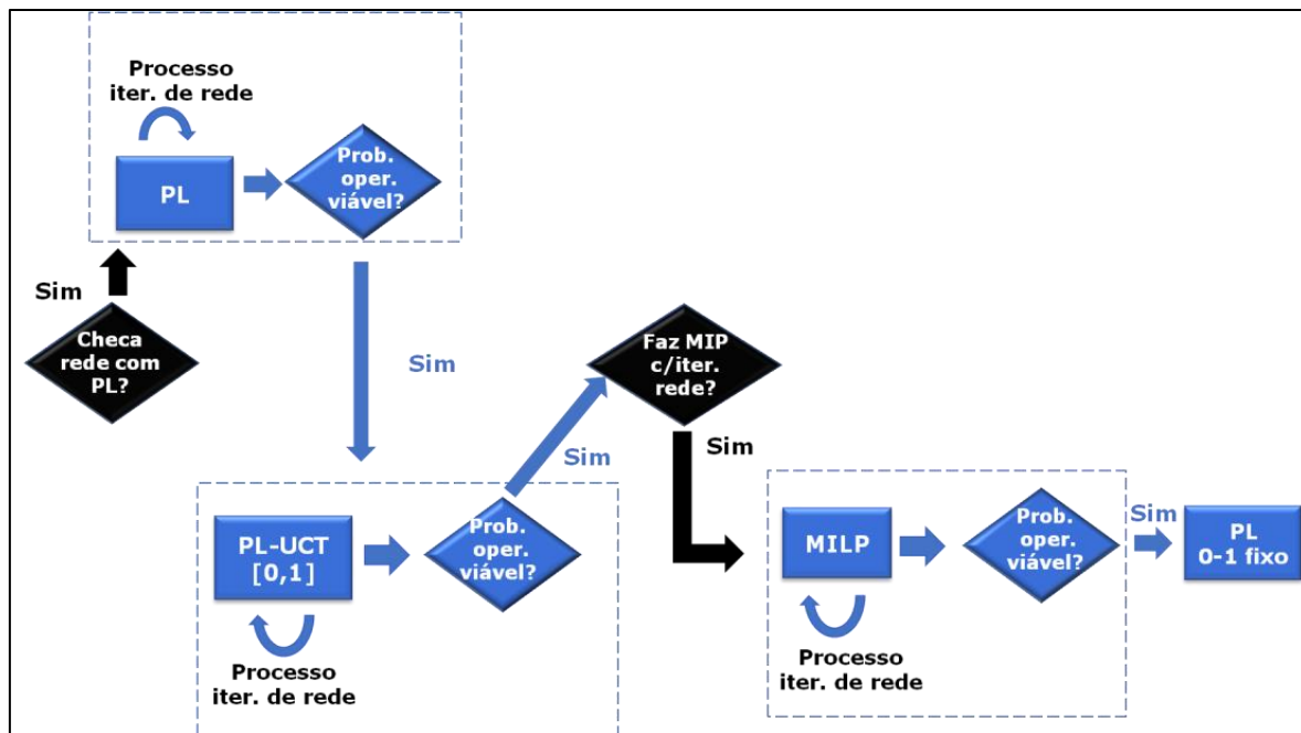
Figura 21-3 - Fluxograma para o processo iterativo com a opção "UCTERM 3".
