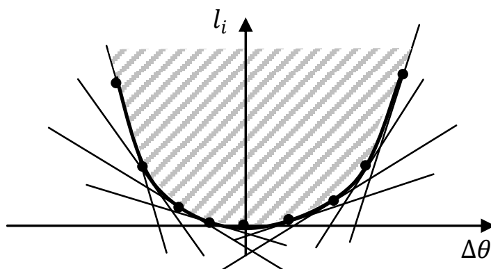
Figura 11-2 - Exemplo de uma aproximação linear por partes para as perdas de transmissão em uma linha i .
