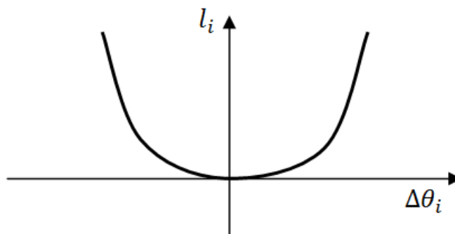
Figura 11-1 - Perdas em um circuito como função quadrática da diferença angular entre suas barras extremas, segundo a modelagem DC com perdas
