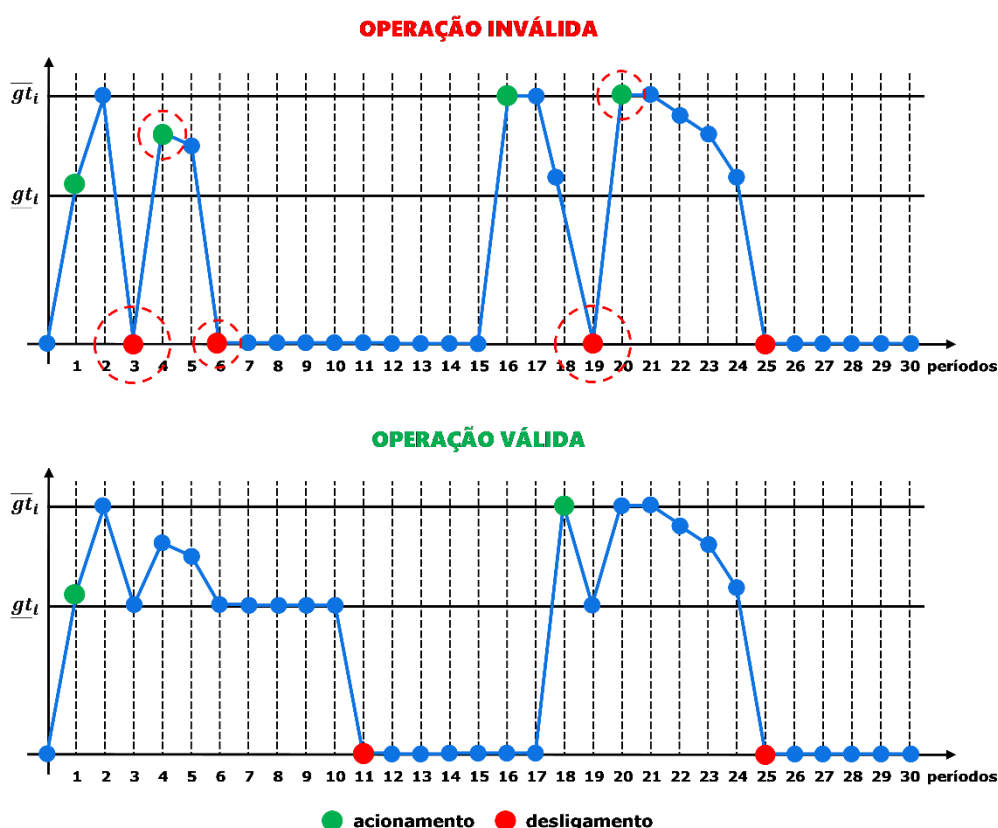
Figura 7-1 - Esquema ilustrativo do efeito das restrições de tempo mínimo ligada/desligada de uma unidade térmica.
