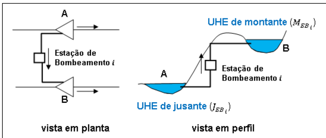
Figura 6-8 - Representação esquemática de uma estação de bombeamento, que transfere água do reservatório A para o reservatório B.
