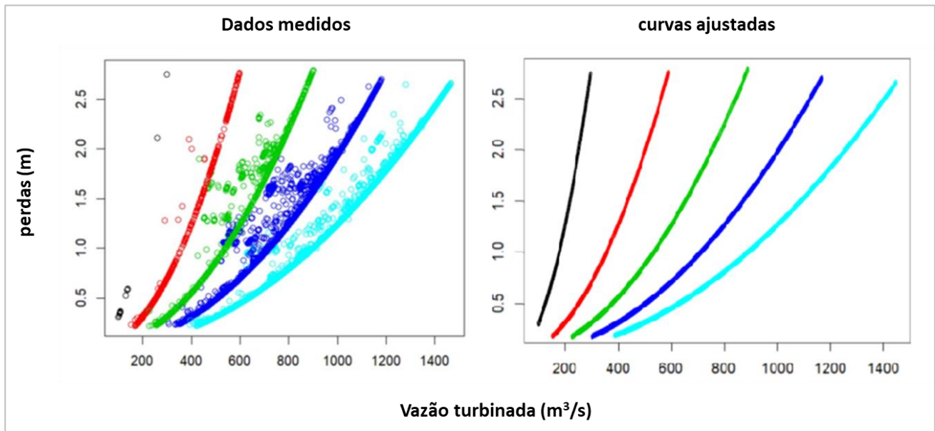
Figura 6-18 – Dados medidos e curva ajustada para as perdas nos conjuntos em função da vazão turbinada da usina.
