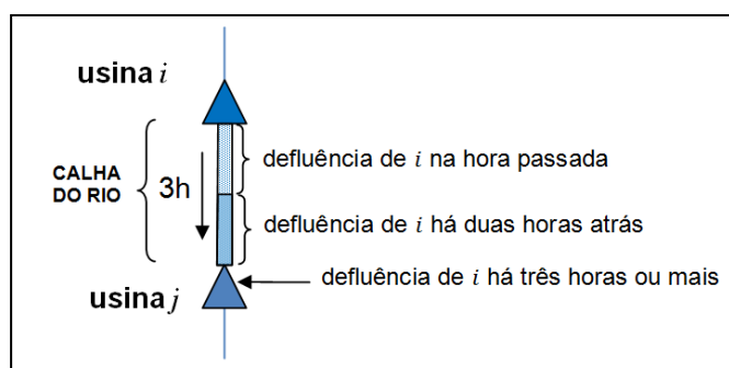
Figura 6-15 - Esquema ilustrativo da água retida na calha do rio para usinas com tempo de viagem da água
