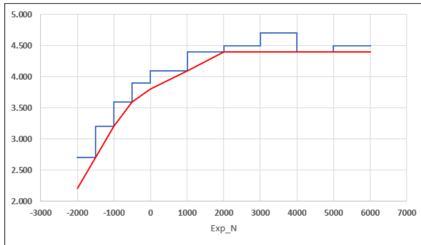
Figura 18-3 - Exemplo de uma restrição de segurança dinâmica da rede elétrica aproximada por uma função linear por partes.
