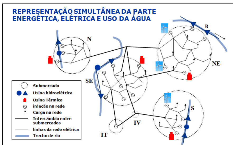
Figura 1-1 – Representação conjunta da rede elétrica, usinas geradoras (hidrelétricas, termoeletrônicas, fontes intermitentes), e trechos de rio no modelo DESSEM.
