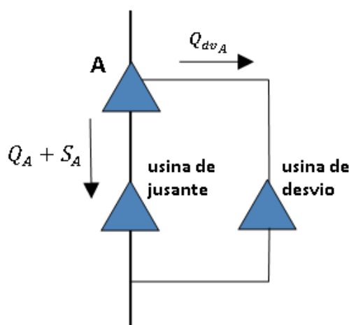
Figura 6-7 - Exemplo ilustrativo de uma usina de desvio.
