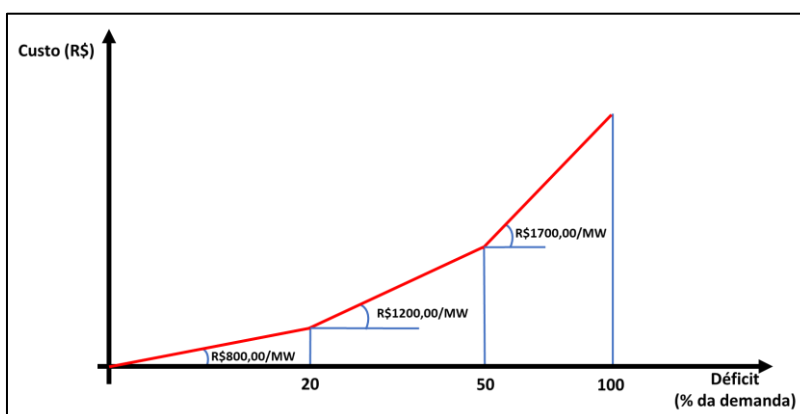
Figura 13-1 - Exemplo de uma curva linear por partes para o custo de déficit de energia.
