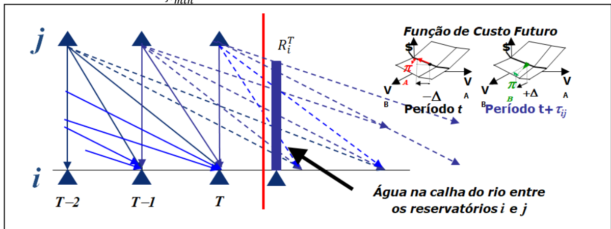
Figura 6-16 - Esquema ilustrativo do acoplamento, com a FCF, das defluências das usinas de montante que ficam na calha do rio ao final do horizonte de estudo.
