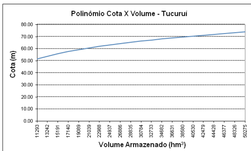
Figura 6-4 - Exemplo do polinômio cota-volume da usina de Tucuruí.
