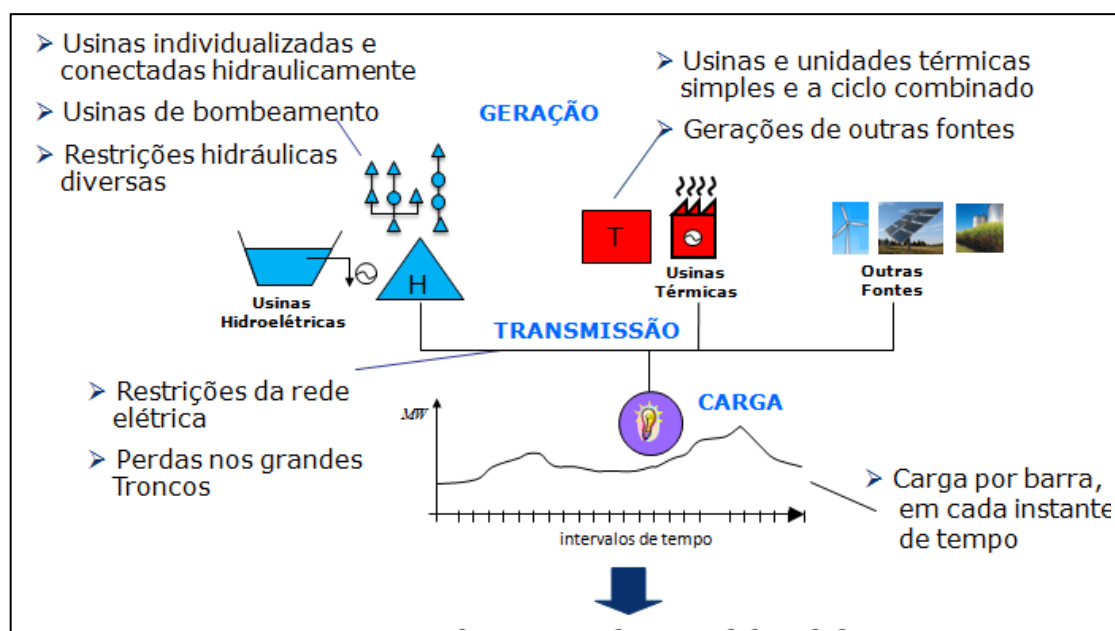
Figura 1-2 - Representação esquemática do problema de programação diária da operação (PDO).
