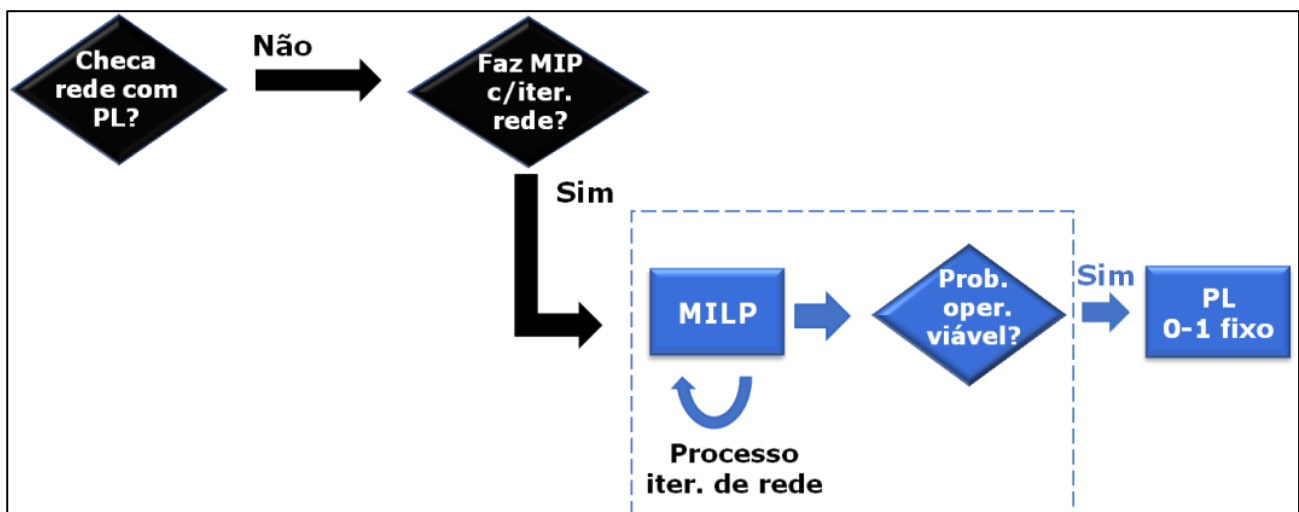
Figura 21-1 - Fluxograma para o processo iterativo com a opção "UCTERM 0".
