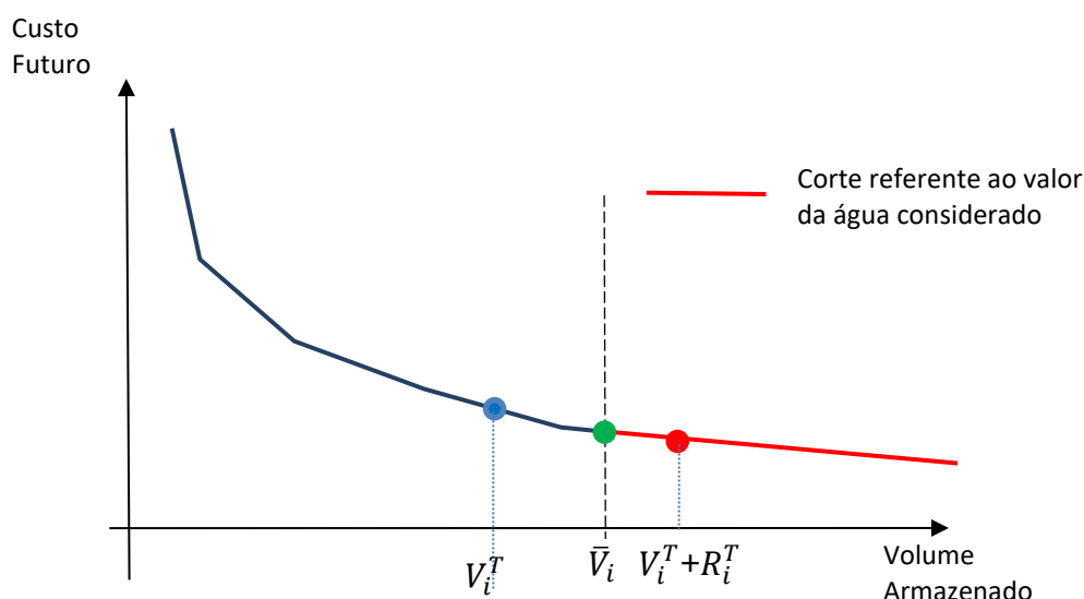
Figura 6.1 - Exemplo de consulta à FCF em um ponto superior ao armazenamento máximo, ao considerar o volume de água na calha do rio.
