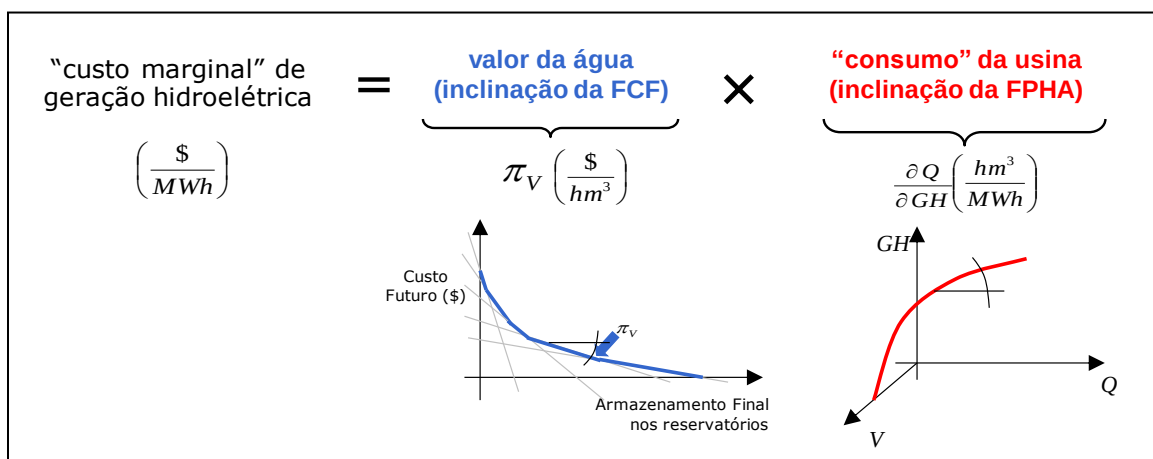
Figura 14-2 - Cálculo implícito do "custo marginal" de geração hidrelétrica, que é realizado implicitamente pelo modelo de coordenação hidrotérmica.
