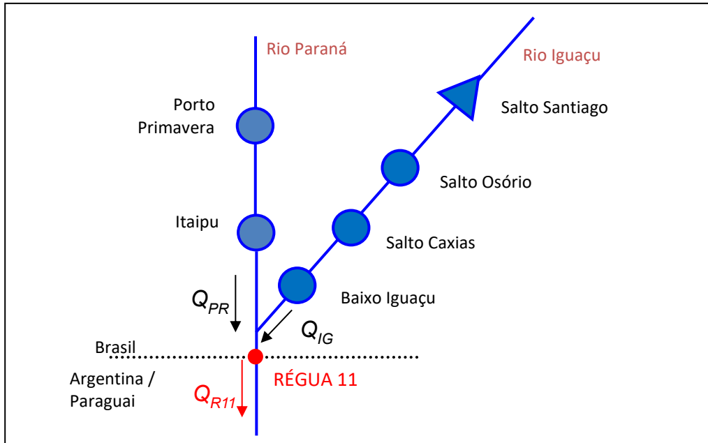
Figura 19-1 - Topologia da cascata à montante da seção da Régua 11.
