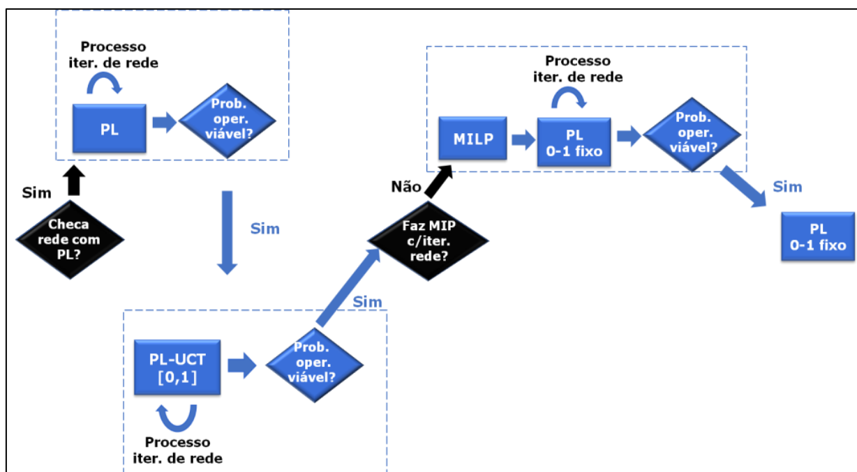
Figura 21-2 - Fluxograma para o processo iterativo com a opção "UCTERM 2".
