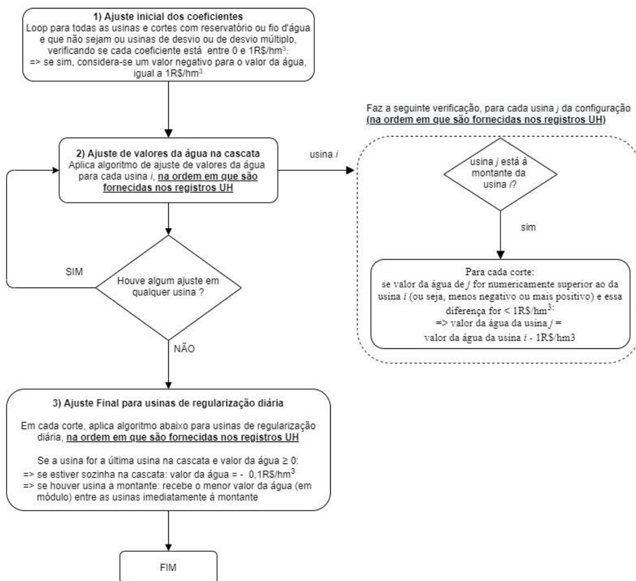
Figura 14-3 - Fluxograma de ajuste nos cortes da FCF do modelo DECOMP, quando se aplica o flag AJUSTEFCF
